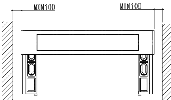
Boven aanzicht
